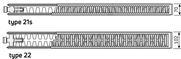
Bovenaanzicht (types 21s & 22) - omkeerbaar
