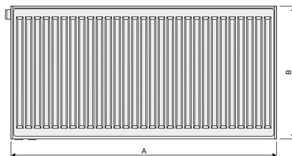
Achteraanzicht (types 21s & 22) zonder ophangstrippen - omkeerbaar
