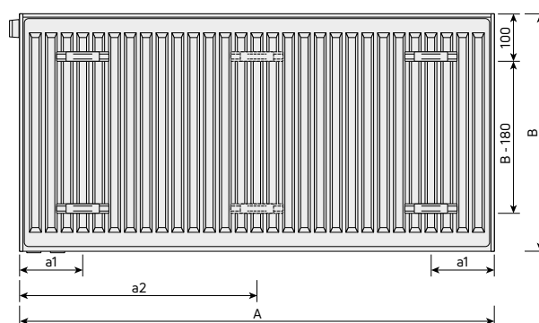
Achteraanzicht (type 33) met ophangstrippen
