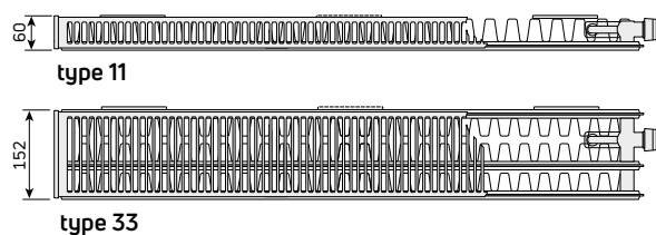
Bovenaanzicht (types 11 & 33)
