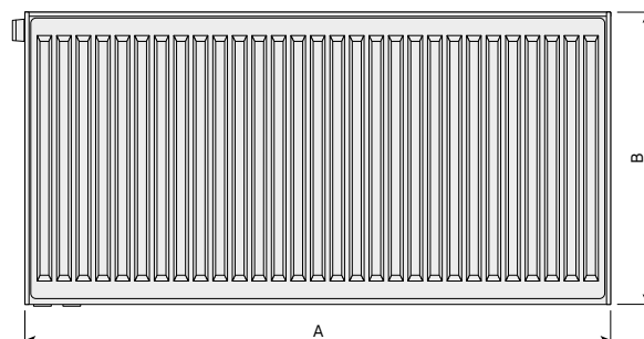
Achteraanzicht (types 21s, 22 & 33) zonder ophangstrippen - omkeerbaar
