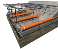
Betonkernactivering
