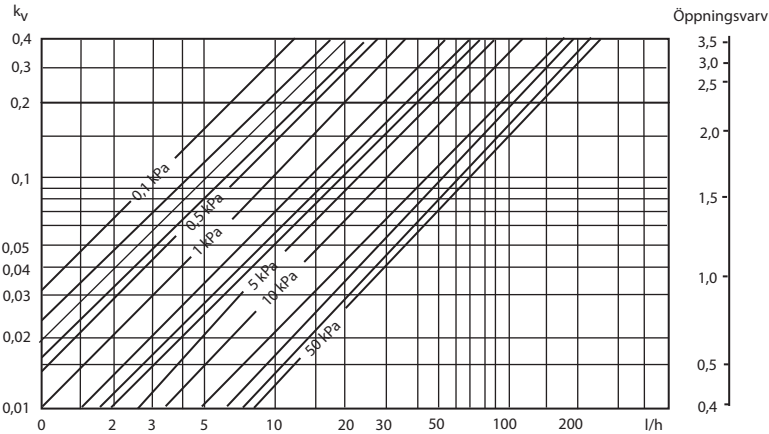
Tryckfallsdiagram för RNT-insats (Thermopanel - ThermoCom)
