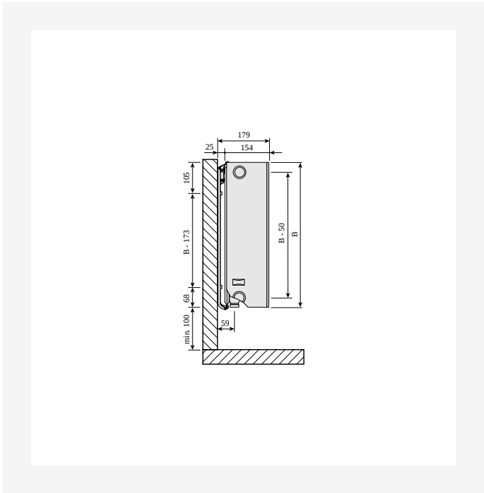
Plan/Ramo/Flex sidovy typ 33
