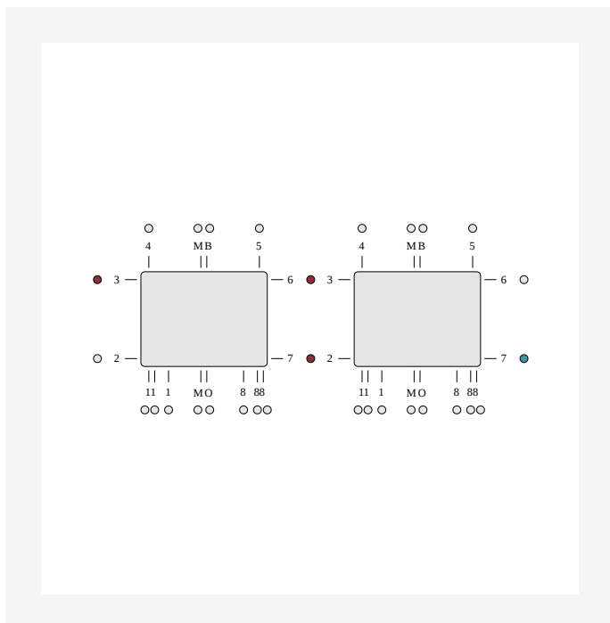
Diagonal seriekoppling vänster ETIM 37
