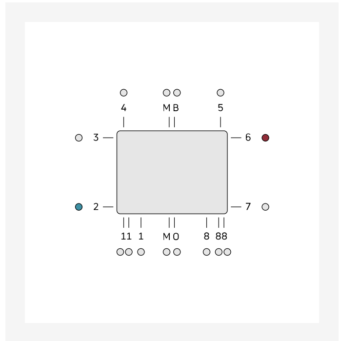
Diagonal anslutning ETIM 62.
