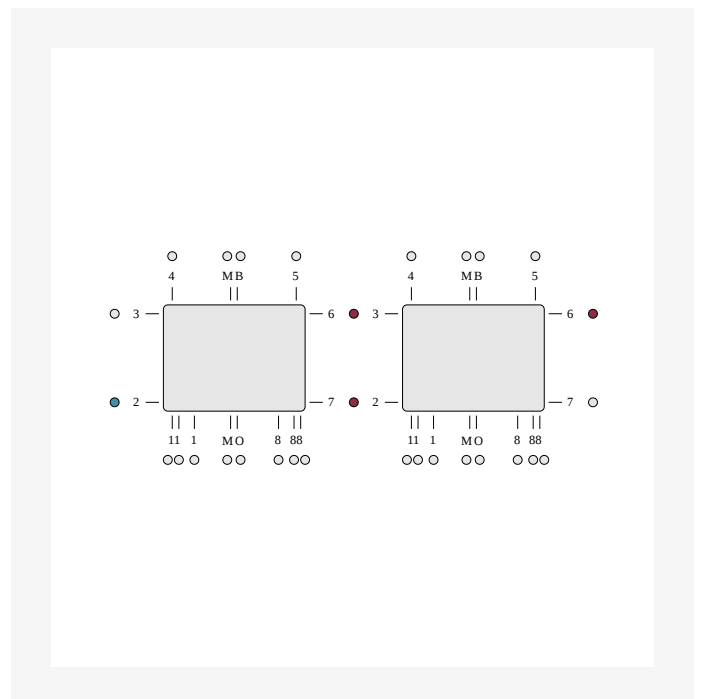
Seriekoppling höger ETIM 62
