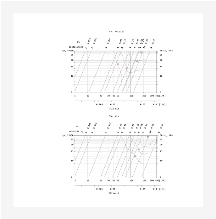
Installationsbild Tryck och flödesdiagram - FLA kvs DT2K
