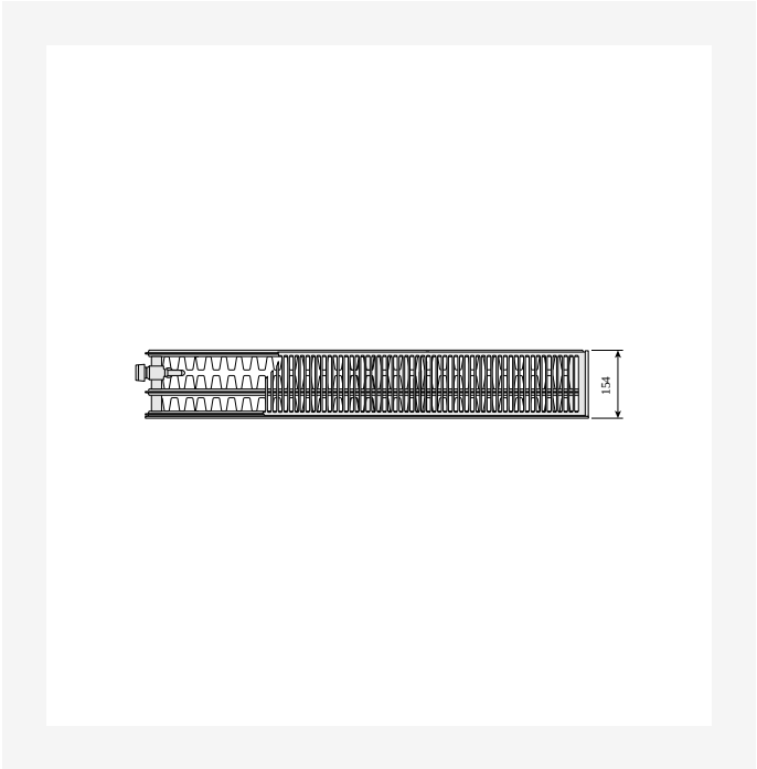
Thermopanel Plan typ 33, vänster toppvy
