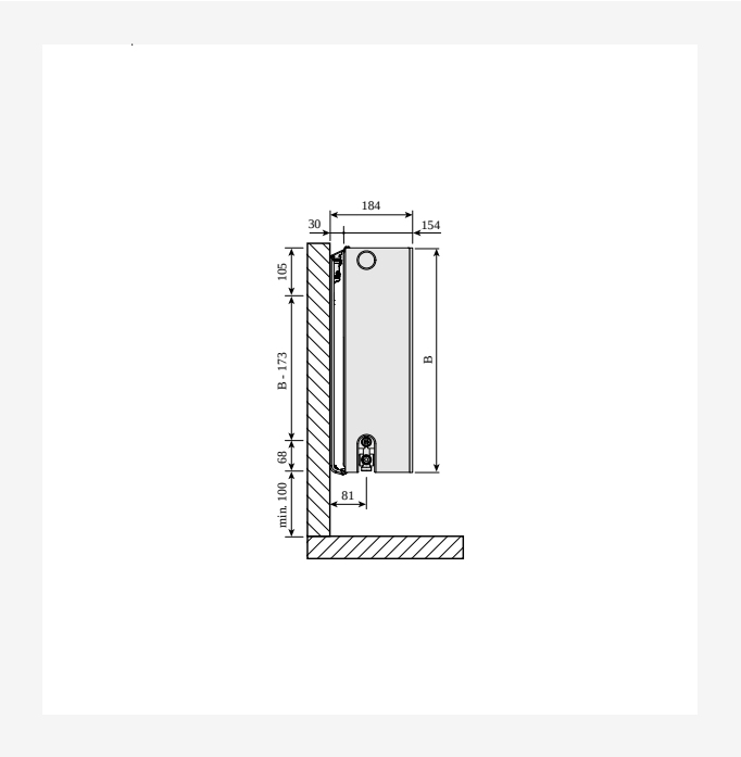
Thermopanel Plan typ 33, sidovy
