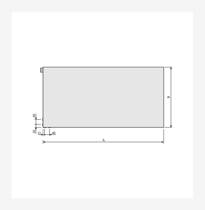
Thermopanel Plan, frontvy vänster
