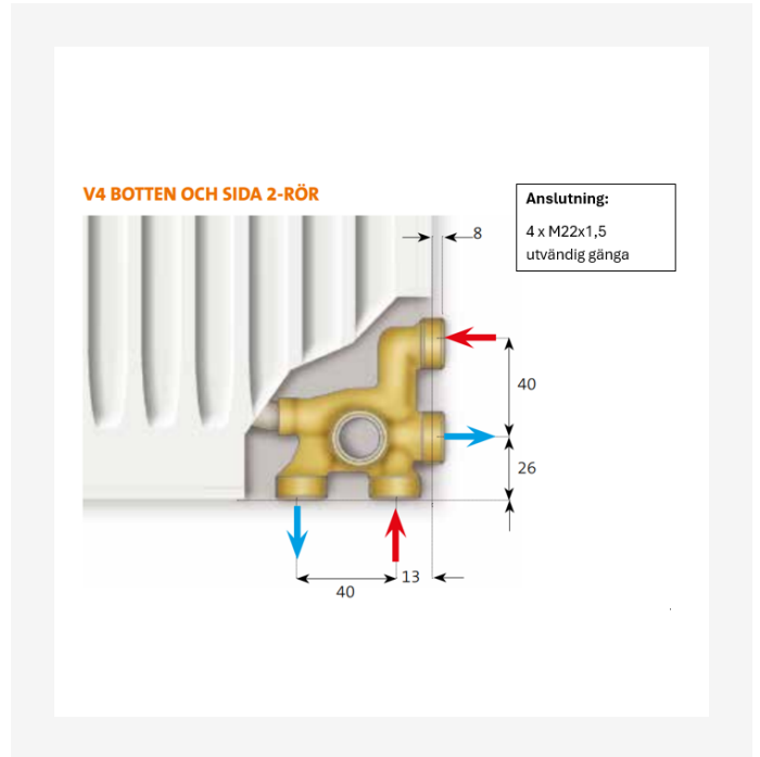
Anslutningsmått TPV4
