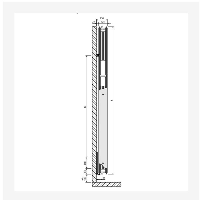
Vertical typ 22, sidovy
