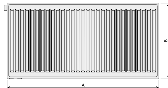
Achteraanzicht (types 21s, 22 & 33) zonder ophangstrippen - omkeerbaar voor types 21s en 22
