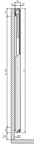
Plan Coté - New_Tinos V-Paros V_SV_T11_0124
