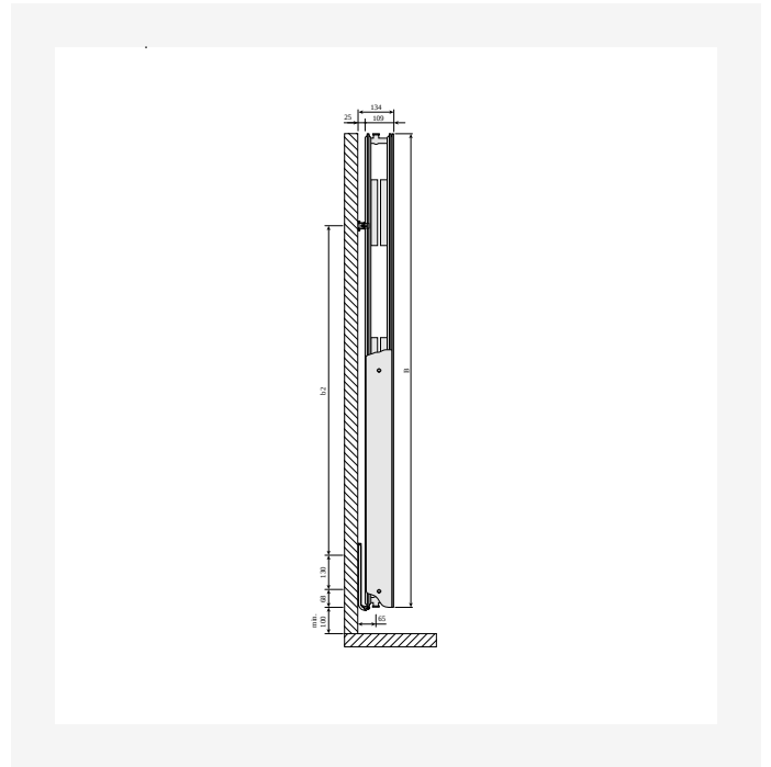
Dimensietekening - PR-KOV-FAV-T22-SV-0120
