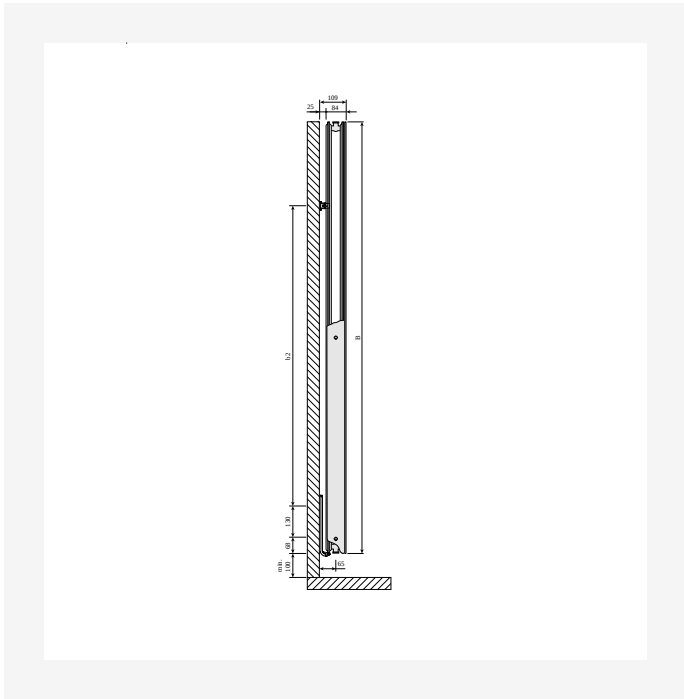
Dimensietekening - PR-KOV-FAV-T20-SV-0120
