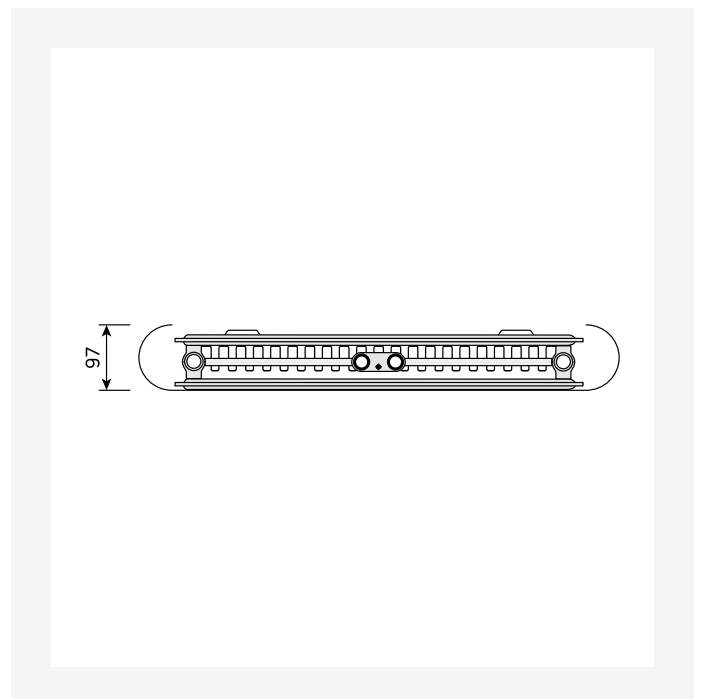
Dimensietekening - New_Paros V_TV_T21_0124
