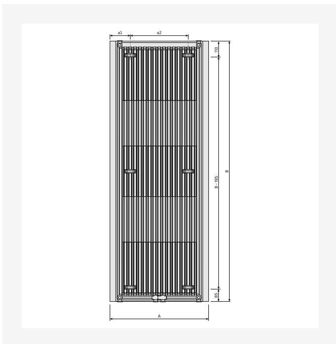
Dimensietekening - New_Paros V_RV_T11_0124
