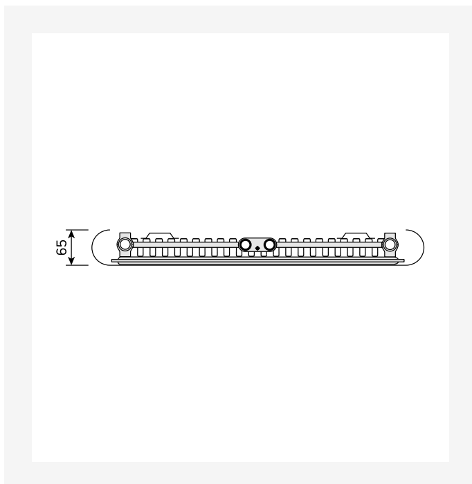
Dimensietekening - New_Paros V_TV_T11_0124
