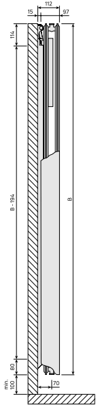
Dimensietekening - New_Tinos V-Paros V_SV_T21_0124
