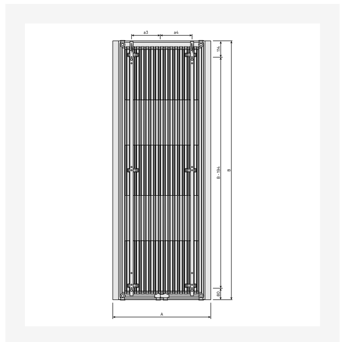
Dimensietekening - New_Paros V_RV_T11_MCWV_0124
