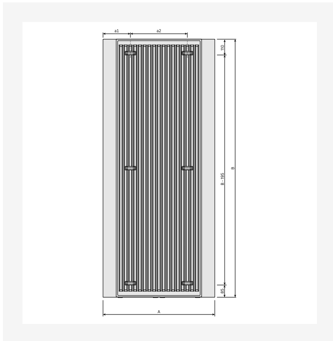
Dimensietekening - New_Paros V_RV_T21_0124
