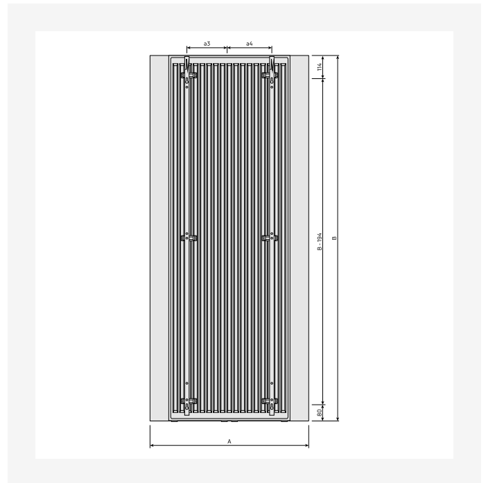
Dimensietekening - New_Paros V_RV_T21_MCWV_0124
