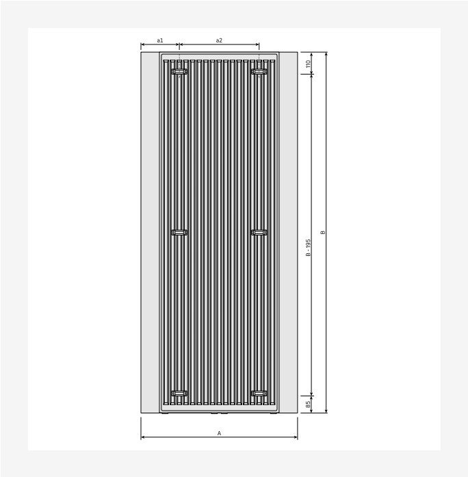
Dimensietekening - New_Paros V_RV_T21_0124
