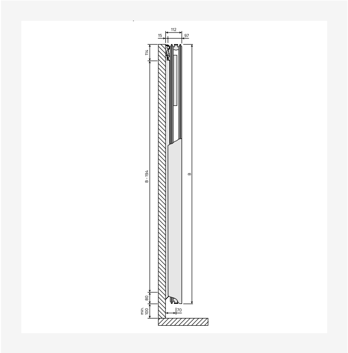
Dimensietekening - New_Tinos V-Paros V_SV_T21_0124
