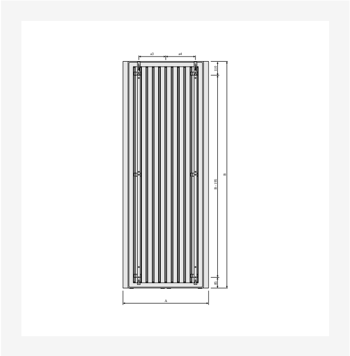
Dimensietekening - PR-PAV-BV-MCW-V-0721
