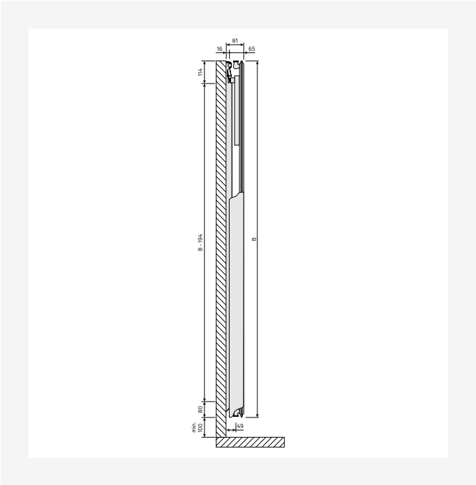
Dimensietekening - New_Tinos V-Paros V_SV_T11_0124
