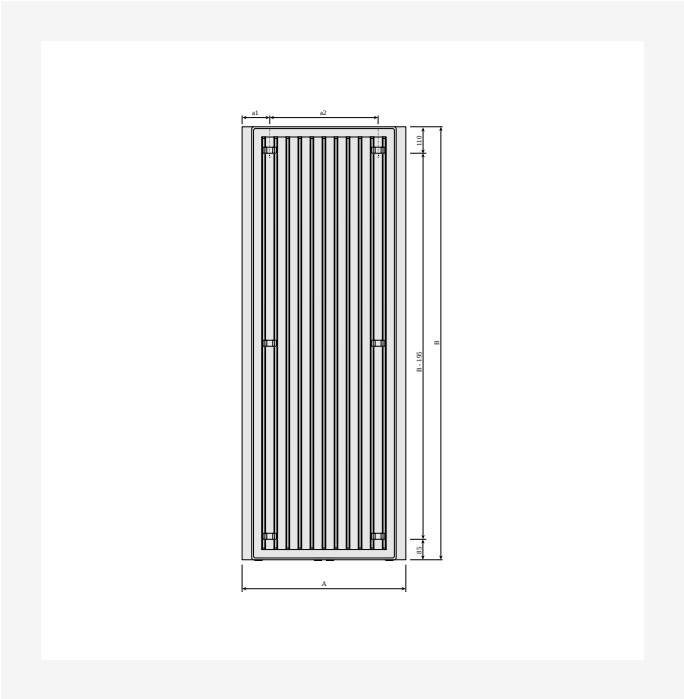
Dimensietekening - PR-PAV-BV-0320
