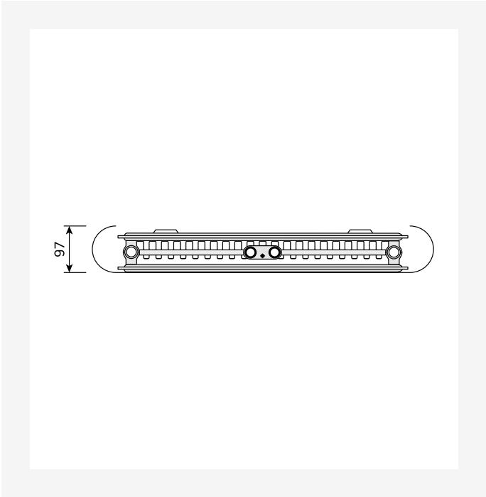
Dimensietekening - New_Paros V_TV_T21_0124
