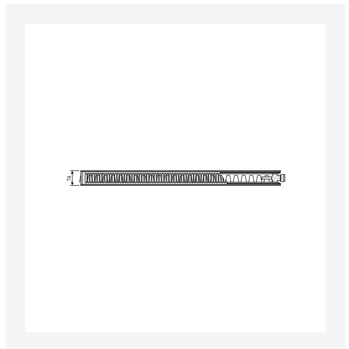
Dimensietekening - PR-Plint-PD-Plint-RD-T21s-TV-0120
