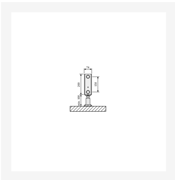
Dimensietekening - PR-Plint-PD-Plint-RD-T21s-SV-Floor-0120
