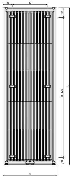
Dimensietekening - New_Tinos V_RV_T11_0124
