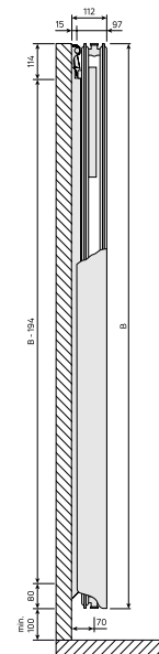
Dimensietekening - New_Tinos V-Paros V_SV_T21_0124
