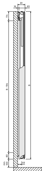
Dimensietekening - New_Tinos V-Paros V_SV_T11_0124
