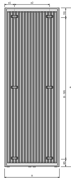
Dimensietekening - New_Tinos V_RV_T21_0124
