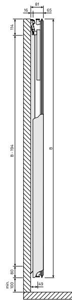
Dimensietekening - New_Tinos V-Paros V_SV_T11_0124
