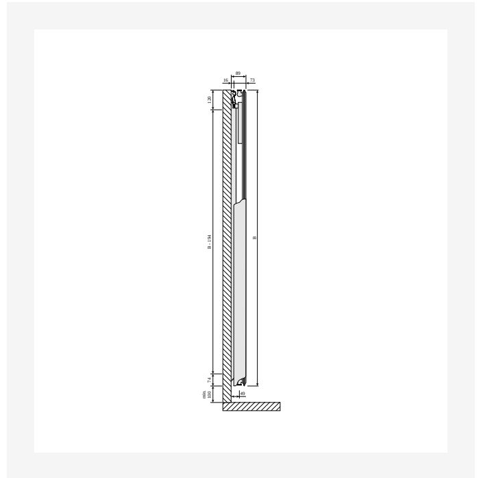
Dimensietekening - PR-TIV-T11-SV-0320
