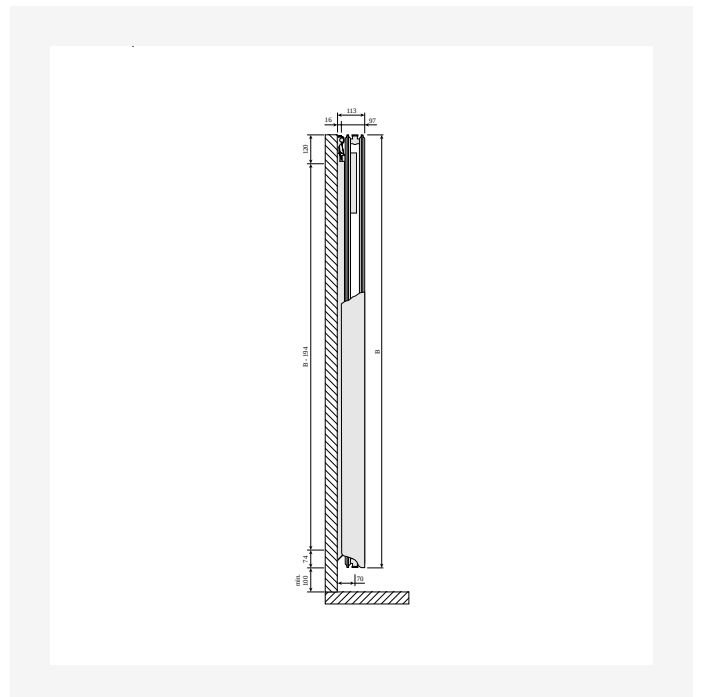
Dimensietekening - PR-TIV-T21-SV-0320
