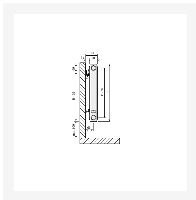
Dimensional Drawing - Compact tyyppi 21, sivukuva SSMS Quick-seinäkiinnikkeillä
