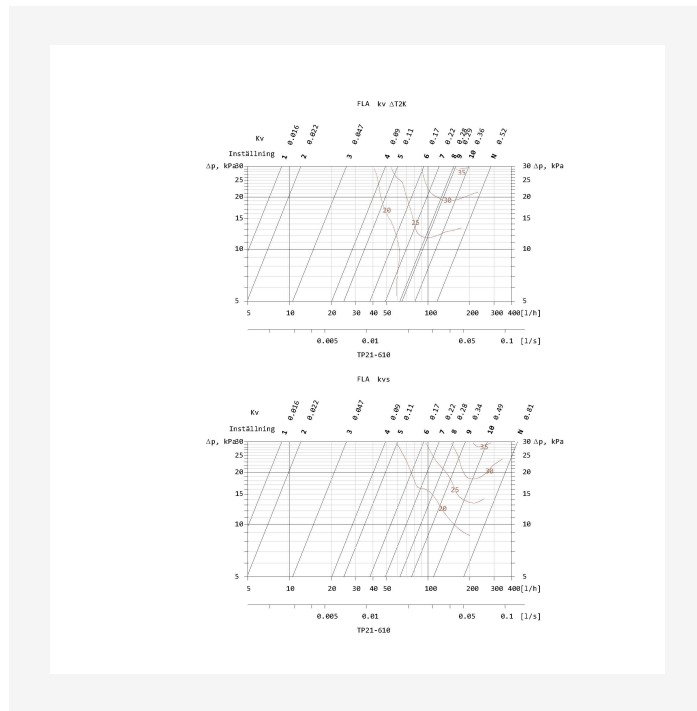
Installation Instructions - FLA-venttiilin kaavio: KVS, KV, \Delta T2K ja äänikäyrä (kuva)
