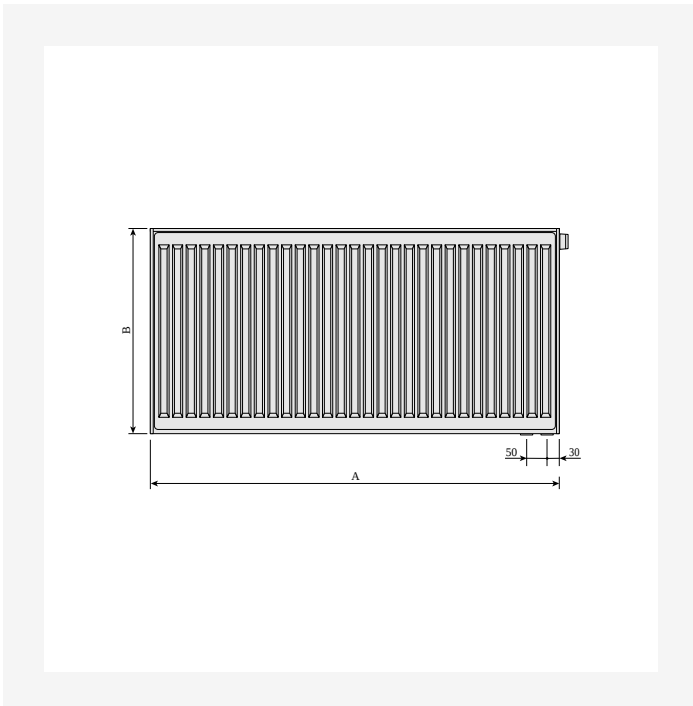
Dimensional Drawing - Ventil Compact, edestä katsottuna
