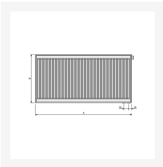
Dimensional Drawing - Ventil Compact, edestä katsottuna
