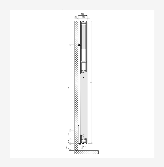
Plan Coté - New_Vertical Vue latérale
