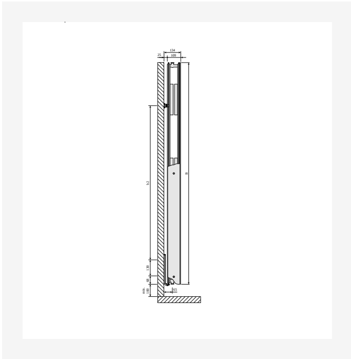
Dimensietekening - PR-KOV-FAV-T22-SV-0120
