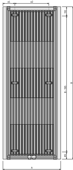
Dimensietekening - New_Paros V_RV_T11_0124
