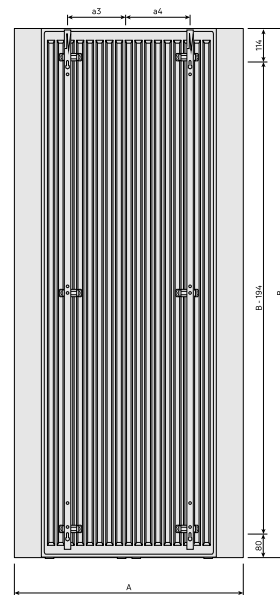
Dimensietekening - New_Paros V_RV_T21_MCWV_0124
