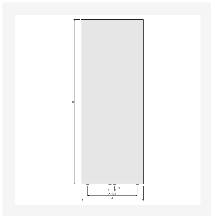
Dimensietekening - New_Paros V_FV_T11_0124
