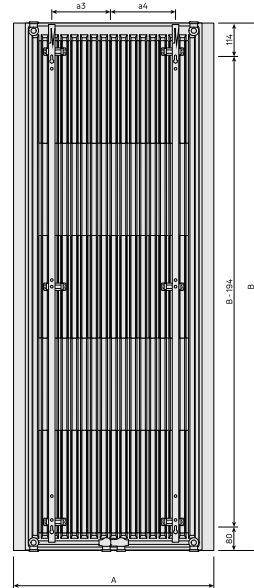
Dimensietekening - New_Paros V_RV_T11_MCWV_0124
