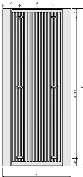
Dimensietekening - New_Paros V_RV_T21_0124
