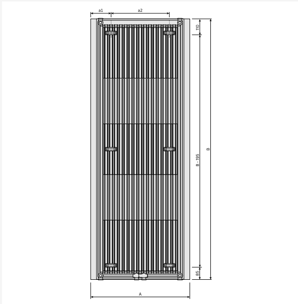
Dimensietekening - New_Paros V_RV_T11_0124
