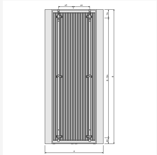
Dimensietekening - New_Paros V_RV_T21_MCWV_0124
