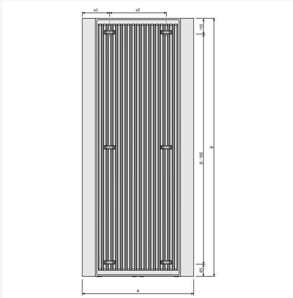
Dimensietekening - New_Paros V_RV_T21_0124
