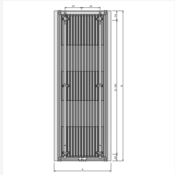
Dimensietekening - New_Paros V_RV_T11_MCWV_0124
