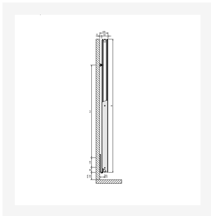
Schiță dimensională - Kos V and Faro V type 20, vedere laterală
