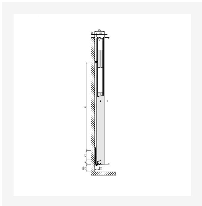
Schiță dimensională - Kos V and Faro V type 22, vedere laterală
