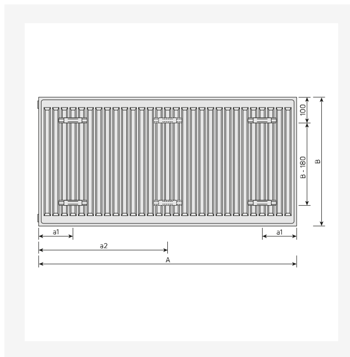
Schiță dimensională - Plan Hygiene, vedere din spate
