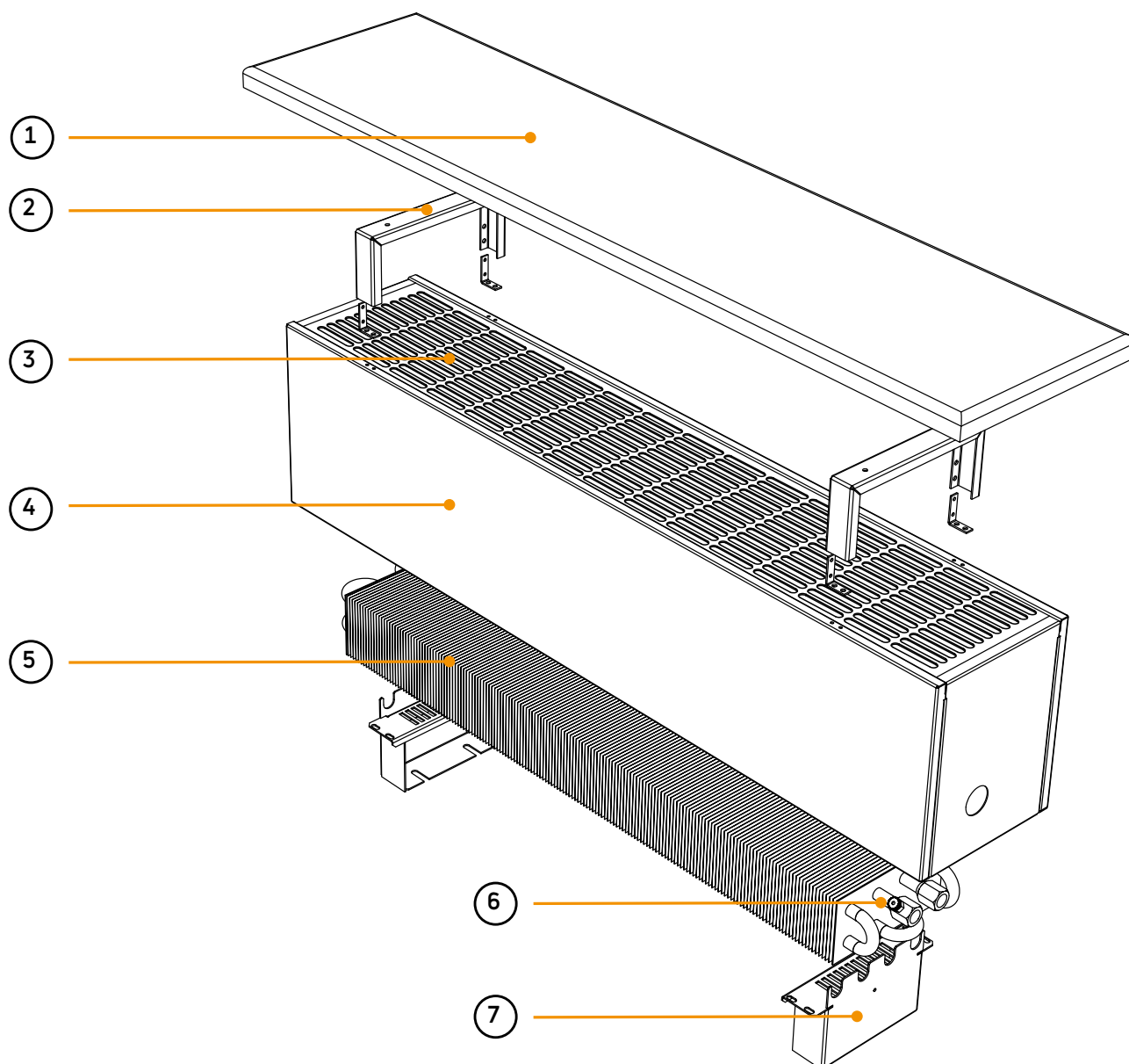
Konstrukcja grzejników Aura Bench WDF
