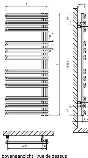
bovenaanzicht | vue de dessus
