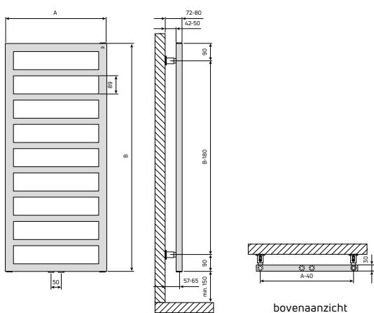
bovenaanzicht
