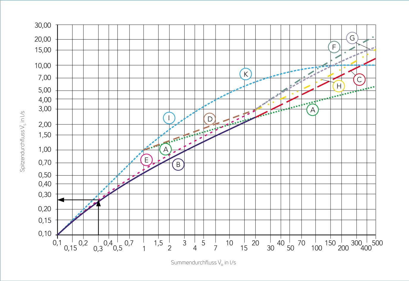
Spitzendurchfluss \dot{V}_s in Abhängigkeit vom Summendurchfluss \dot{V}_R (Auszug aus DIN 1988/Teil 3 ,Bild 3)
