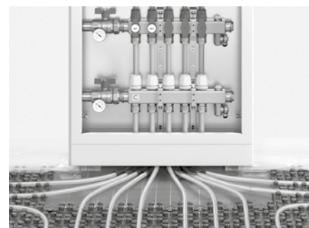
Abb. 6: Heizrohr am Verteiler anbringen, fertig!
