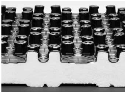
Abb. 3: Noppenplatte 30-2 mm
