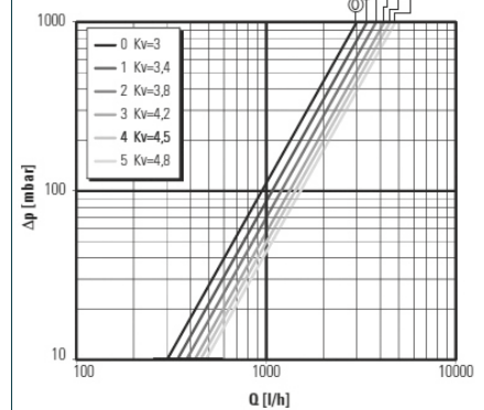
Druckabfalldiagramm
