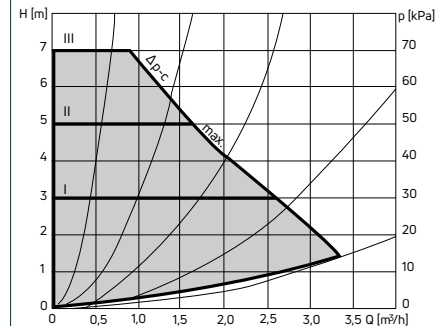
Pumpendiagramm
