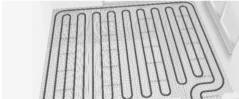
Abb. 1: mäanderförmige Verlegung
